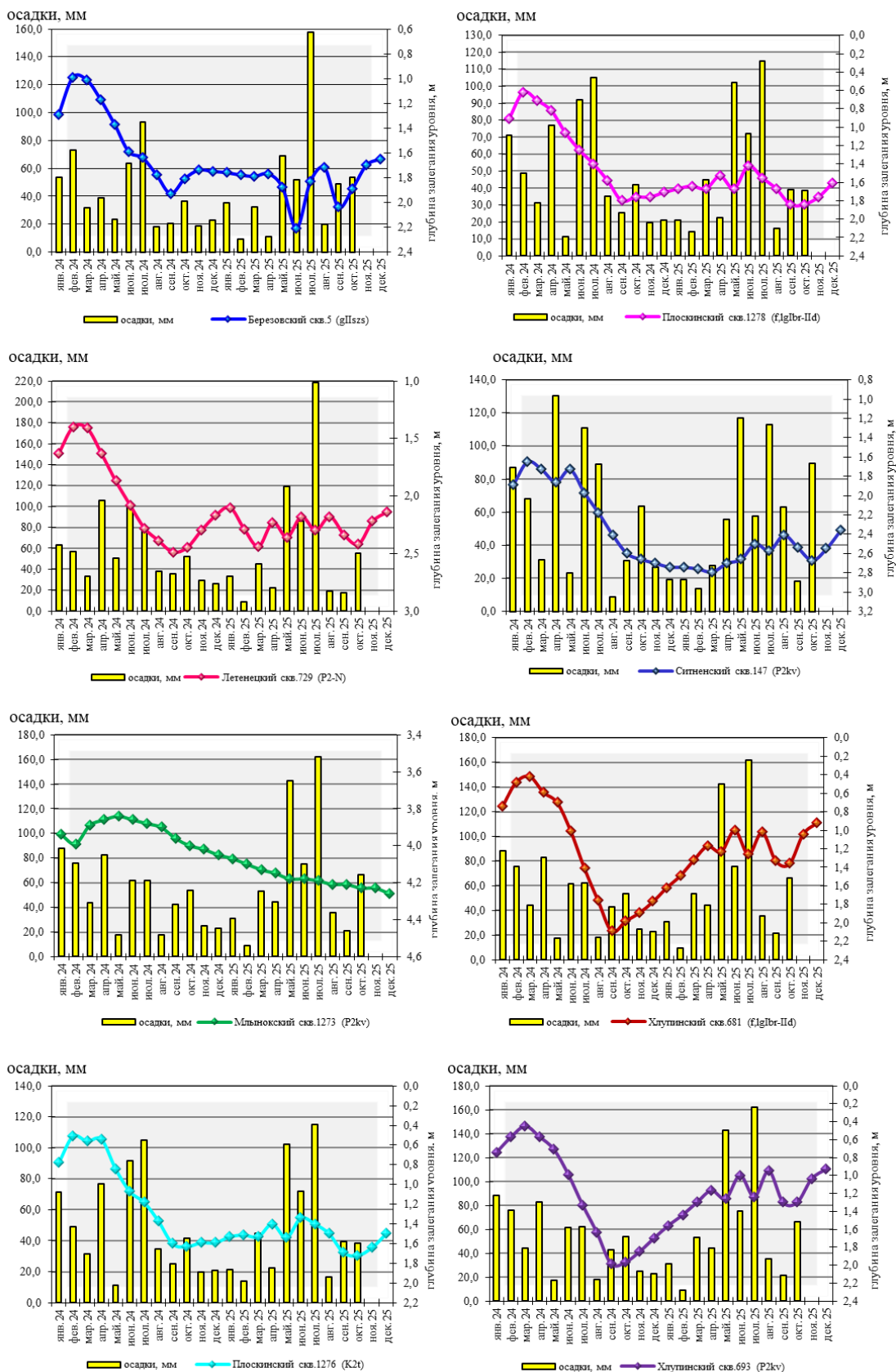
Рисунок 3.18 – Графики изменения сезонного режима уровней артезианских вод в бассейне р. Припять
