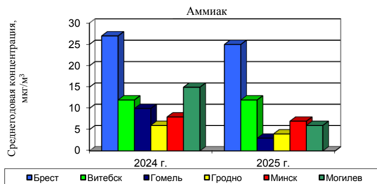
Рисунок 4.43 – Концентрации аммиака в атмосферном воздухе областных центров Республики Беларусь в 2024 – 2025 гг.
