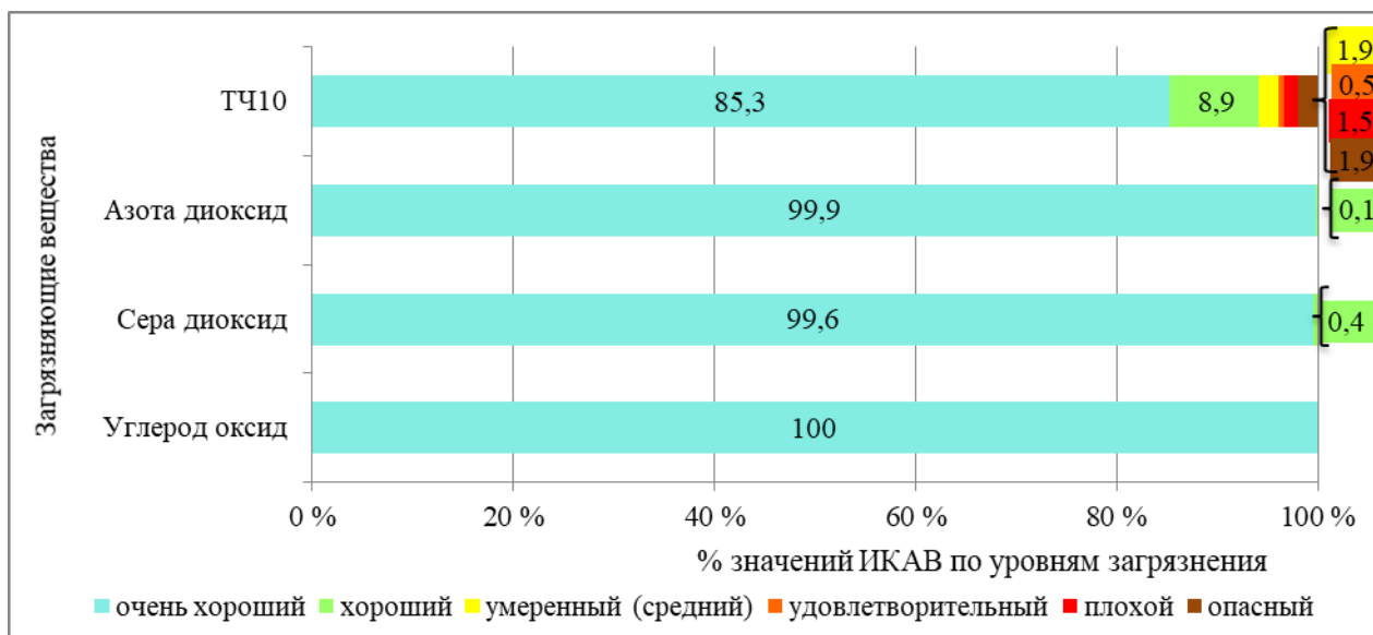
Рисунок 4.82 – Распределение значений ИКАВ (%) в 2025 г. в г. Сморгонь (район ул. Корени, 48А)
