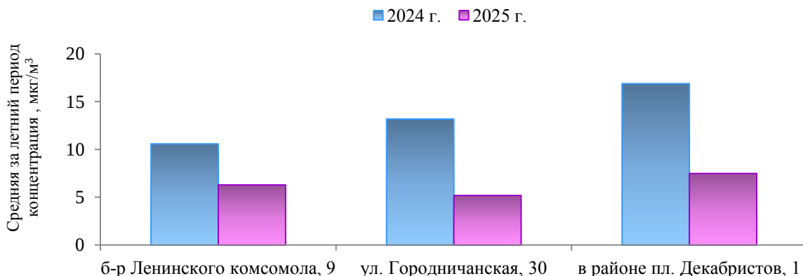
Рисунок 4.26 – Средние за летний период концентрации формальдегида в атмосферном воздухе г. Гродно, 2024 – 2025 гг.
