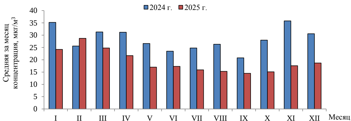
Рисунок 4.63 – Внутригодовое распределение среднемесячных концентраций серы диоксида в атмосферном воздухе г. Новополюцк по данным наблюдений на пунктах с дискретным режимом отбора проб, 2024 – 2025 гг.
