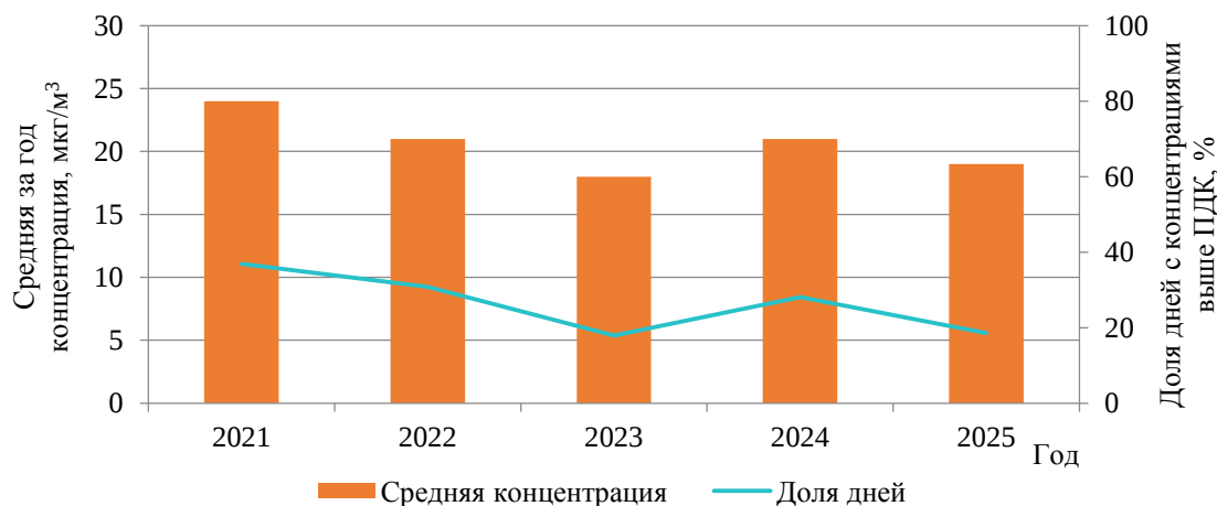
Рисунок 4.33 – Средние за год концентрации ТЧ 2,5 и доля дней с концентрациями выше ПДК в воздухе г. Жлобин (район ул. Пригородная, д. 12) в 2021 – 2025 гг.
