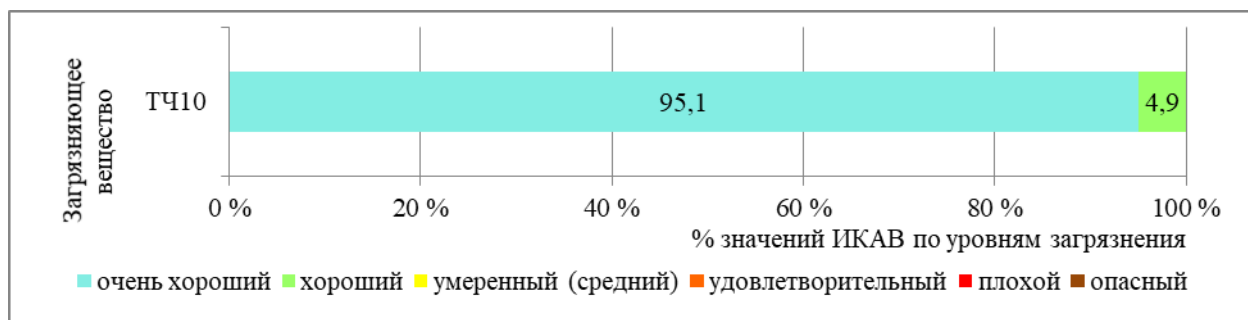
Рисунок 4.48 – Распределение значений ИКАВ (%) в 2025 г. в г. Могилев (район ул. Мовчанского, 4)
