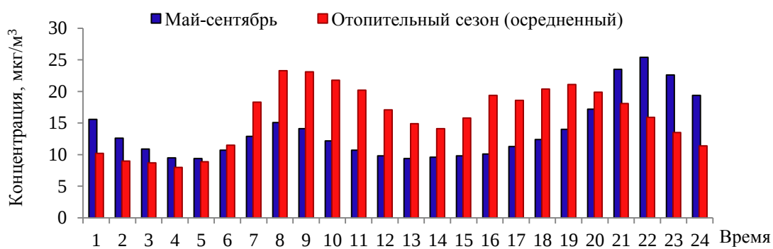
Рисунок 4.42 – Суточный ход концентраций азота диоксида, г. Минск, микрорайон «Уручье», 2025 г.
