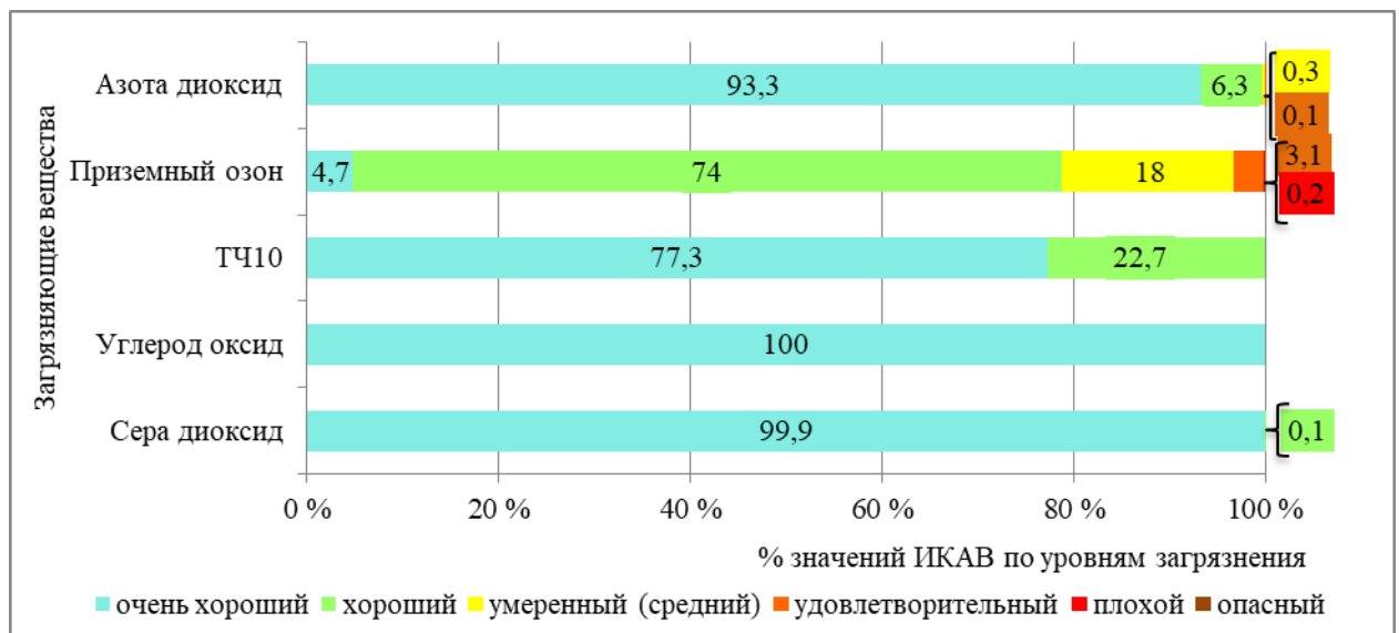
Рисунок 4.62 – Распределение значений ИКАВ (%) в 2025 г. в г. Новополоцк (район административного здания по улице Молодежная, 49, корпус 1)
