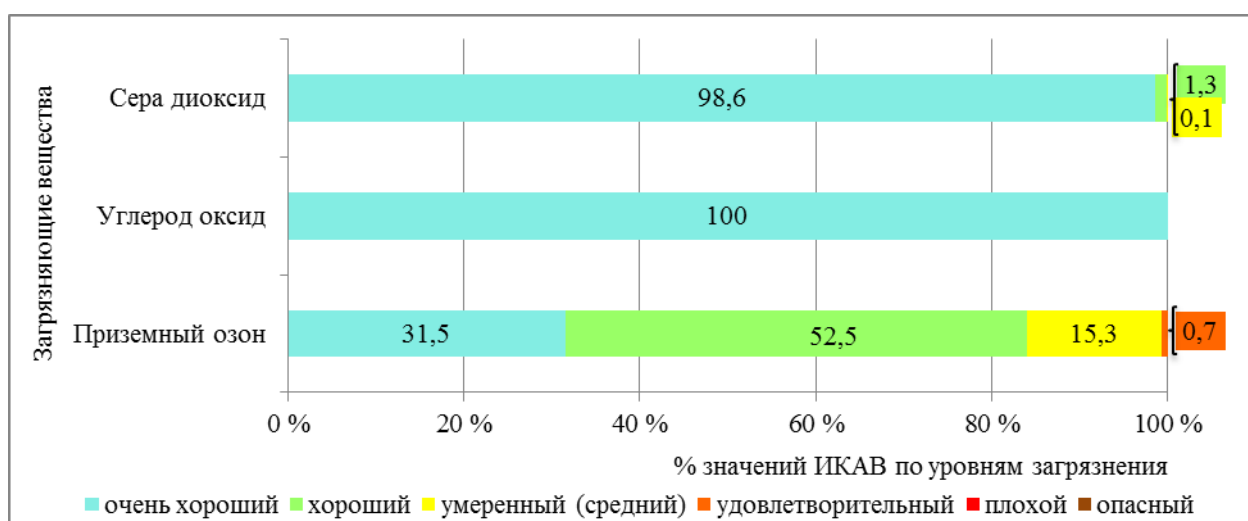
Рисунок 4.56 – Распределение значений ИКАВ (%) в 2025 г. в д. Пеньки (Мозырский район)
