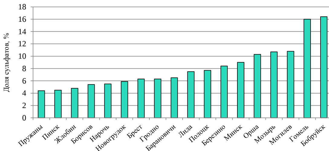
Рисунок 4.90 – Доля сульфатов в общей минерализация атмосферных осадков в 2025 г.
