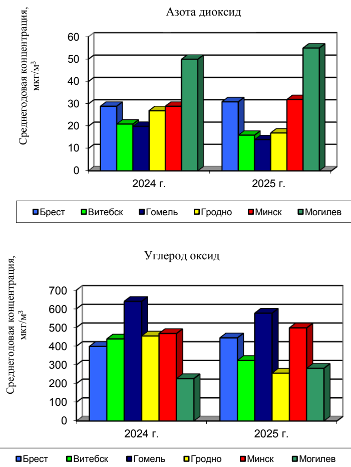
Рисунок 4.41 – Среднегодовые концентрации азота диоксида и углерод оксида в атмосферном воздухе областных центров Республики Беларусь в 2024 – 2025 гг.
