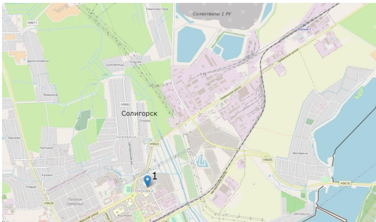
Рисунок 4.85 – Местоположение пунктов наблюдений мониторинга атмосферного воздуха в г. Солигорск
