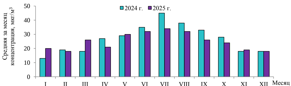
Рисунок 4.10 – Внутригодовое распределение концентраций аммиака в атмосферном воздухе г. Брест в 2024 – 2025 гг.
