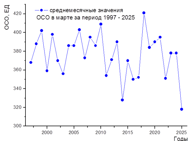
Рисунок 5.2 – Среднемесячные значения ОСО в марте за период 1997 – 2025 гг. (г. Минск)
