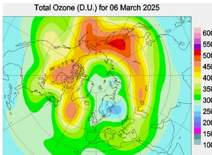
Рисунок 5.3 – Распределение полей ОСО 6 марта 2025 г. Рядом представлена цветовая шкала ОСО
