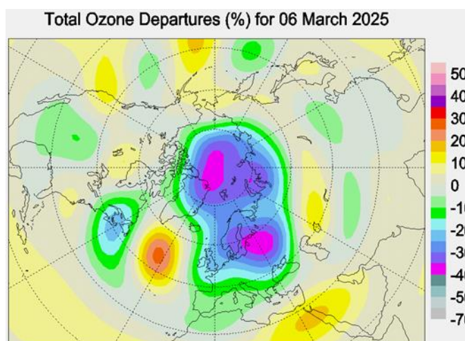
Рисунок 5.4 – Распределение отклонений полей ОСО 6 марта 2025 г. от многолетних средних значений. Рядом представлена цветовая шкала отклонений ОСО в %
