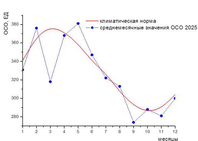
Рисунок 5.1 – Годовой ход ОСО в 2025 г. и климатическая норма для Республики Беларусь (г. Минск)
