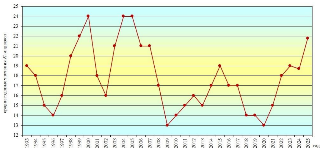
Рисунок 9.8 – График долговременных вариаций среднегодовых значений суммарных K -индексов за 1993 – 2025 гг.
