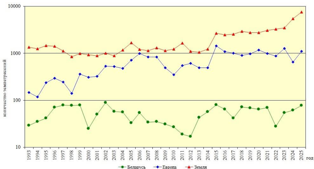
Рисунок 9.18 – График временного хода числа землетрясений на территории Земли, Европы и Республики Беларусь за период 1993 – 2025 гг.
