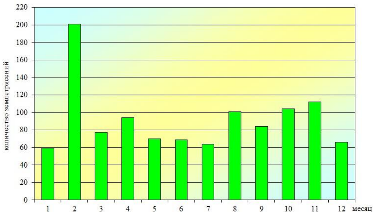
Рисунок 9.16 – График изменения количества землетрясений Европы и смежных областей в 2025 г.
