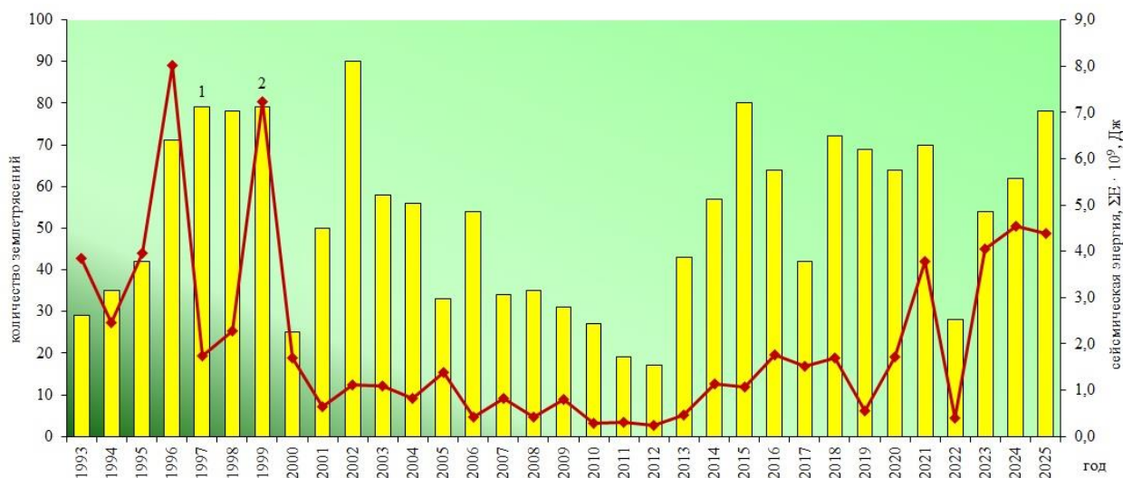
Рисунок 9.4 – График изменения числа сейсмических событий (1) и величины их суммарной сейсмической энергии (2) за 1993 – 2025 гг.
