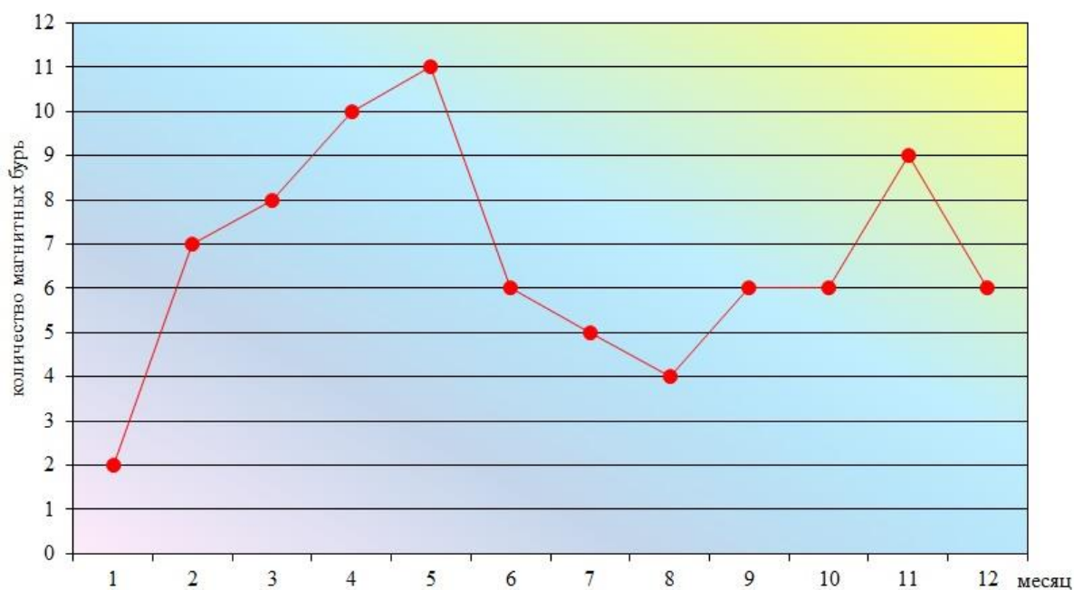
Рисунок 9.10 – График изменения числа магнитных бурь в 2025 г.
